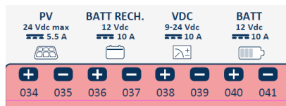
Figura 2.3: morsettiera degli ingressi di alimentazione.
