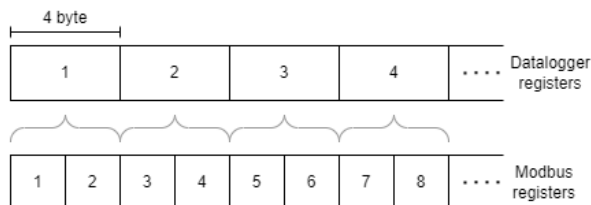
Figura 8.1: corrispondenza tra registri del datalogger e registri Modbus.
