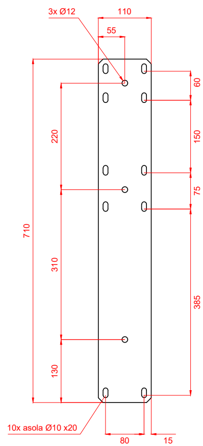
Particolari ingranditi di p099-05 / magnified details of p099-05
