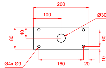
Particolari ingranditi della piastra saldata magnified details of welded plate
