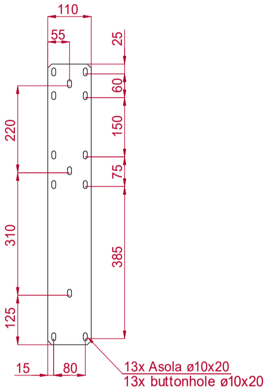
Particolari ingranditi di p099-05 / magnified details of p099-05
