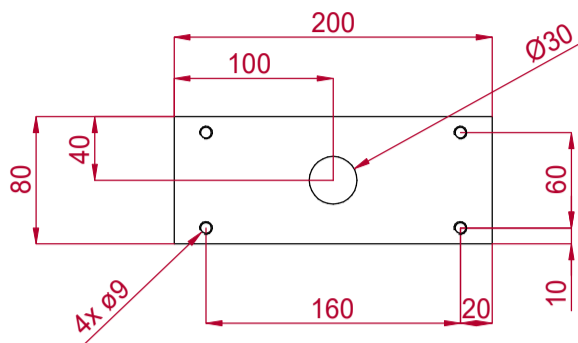
Particolari ingranditi della piastra saldata / magnified details of welded plate
