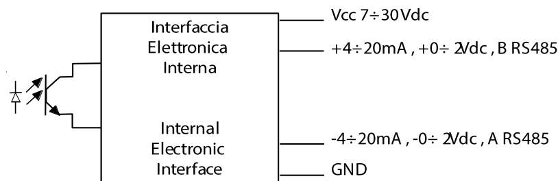
TVV-IVS / TVV-I/V/S Versione con uscita 4÷20mA, 0÷2Vdc, RS485
